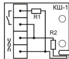
Плата Контроля Шлейфа-1
